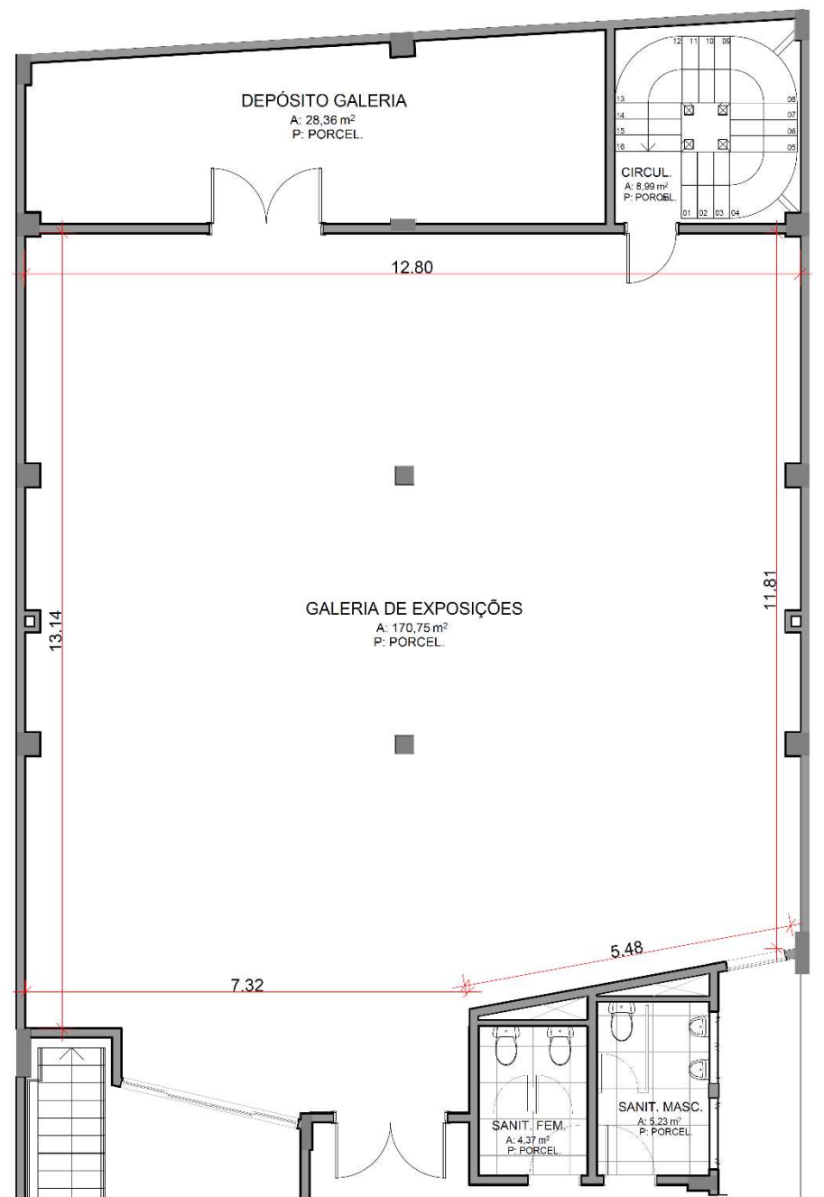
PLANTA BAIXA - TÉRREO ESC: 1/100
